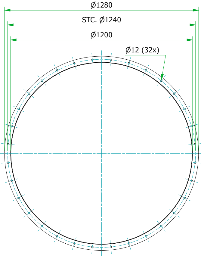
Aanzicht A (1:15)
