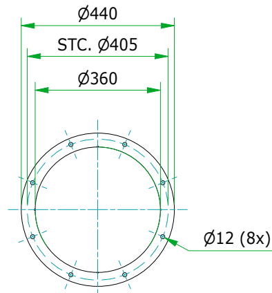
Aanzicht B (1:15)
