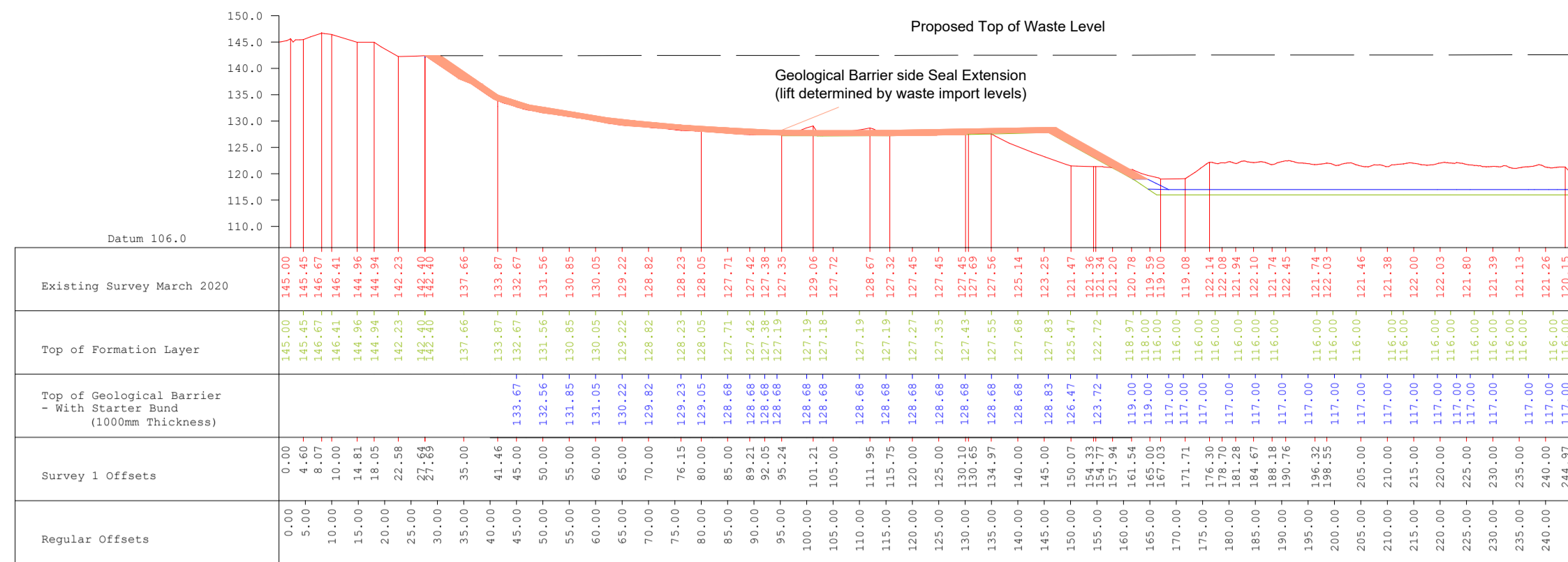
Section A-A' 1:1000
